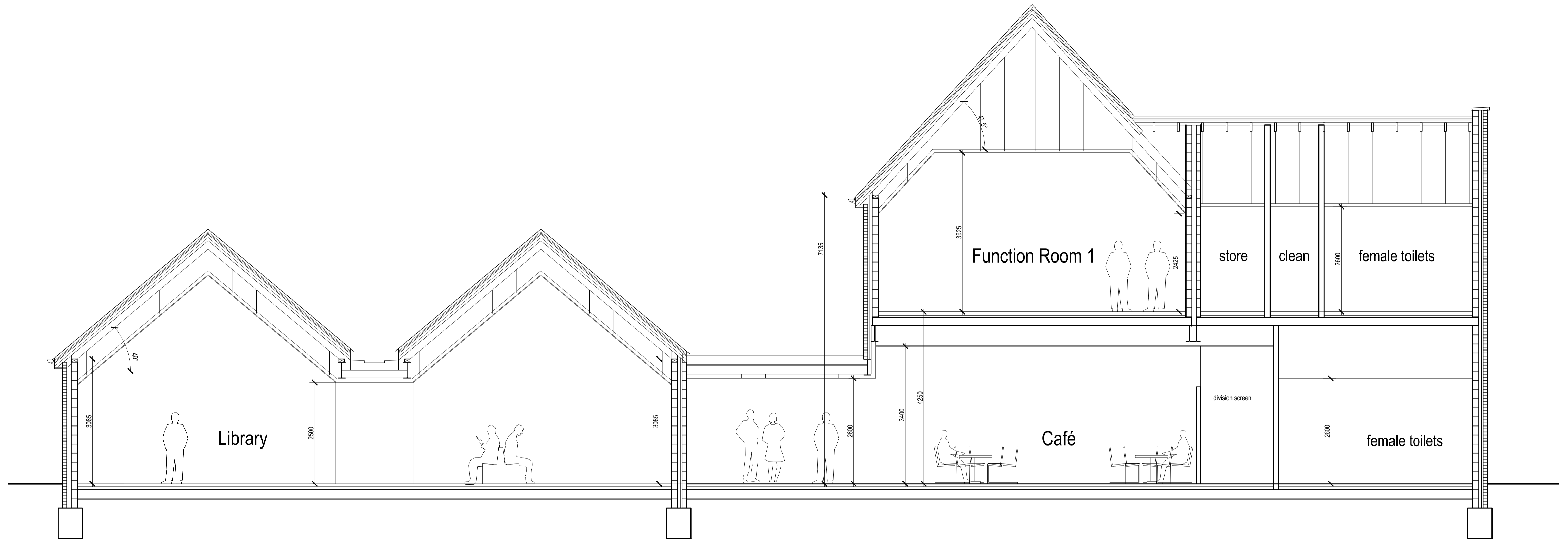
Section A-A
